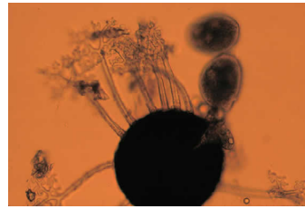
Cleistothecia
